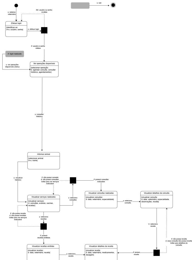
Diagrama MoLIC do objetivo: Consultar histórico - MVP1-MoLIC-2.drawio.png
